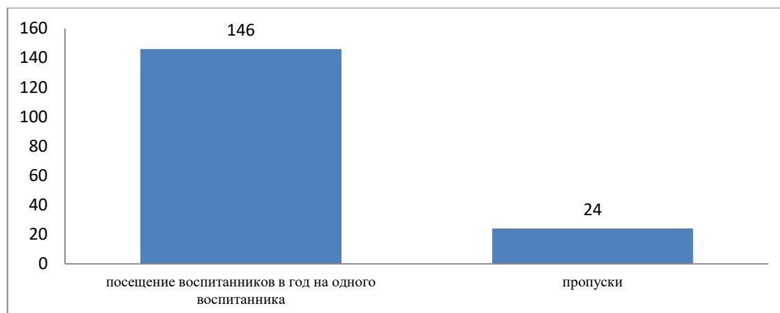
Гистограмма 2.
